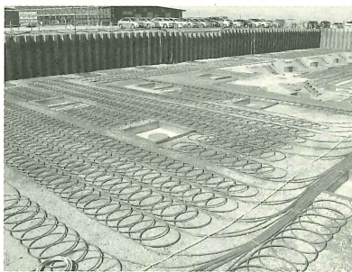
地中熱回収システムのコイル
